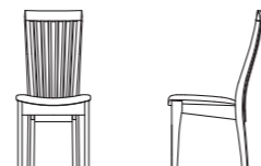
4870 チェア W:446×D:576×H:957 SH:425 才数:12.2 ※ ¥56,500+tax
